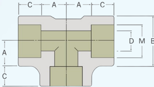
Tee
